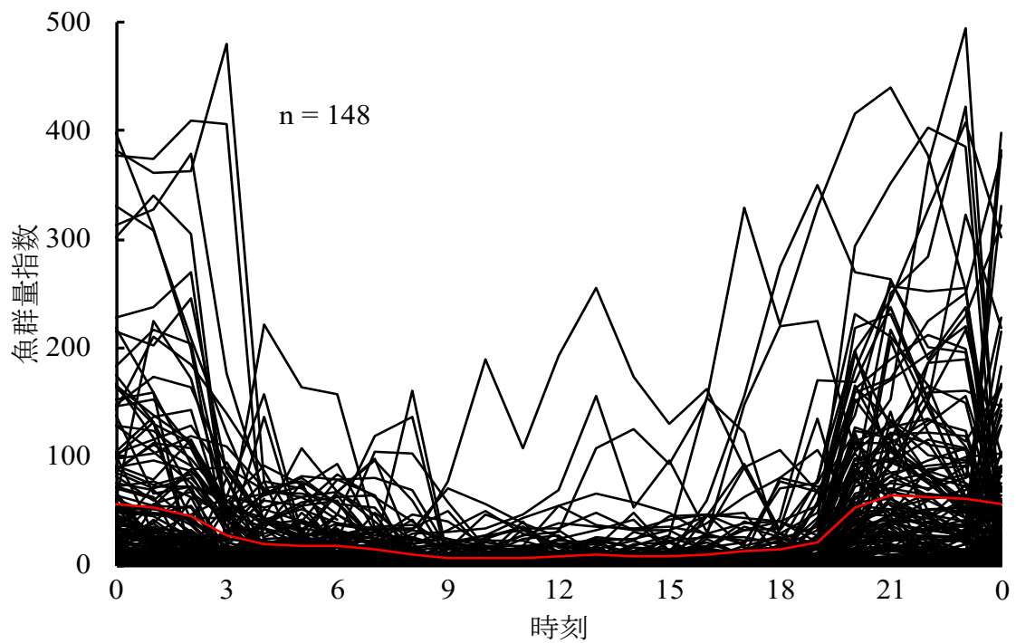
Fig.26 魚群量指数の日周変動
