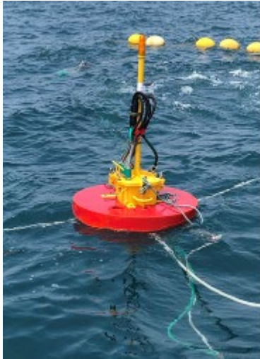
Fig.6 定置網用魚群探知機の海上ブイ(左)と送受波器(右)
