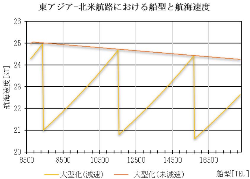
図 5.2.1.9 大型化による隻数増加の減速航海
