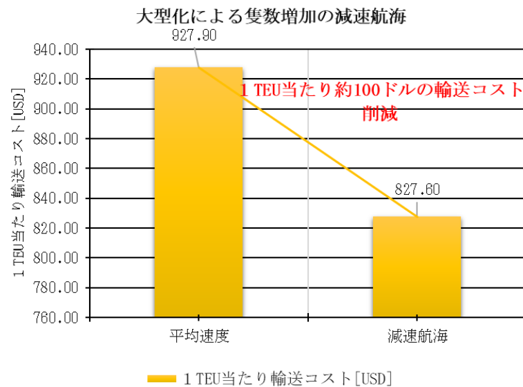
図 5.2.1.7 輸送コストの削減効果 (7,424TEU)
