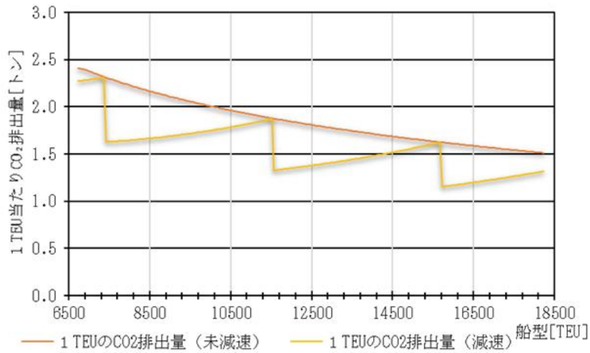
東アジア-北米航路における船型と1TEU当たりCO 2 排出量
