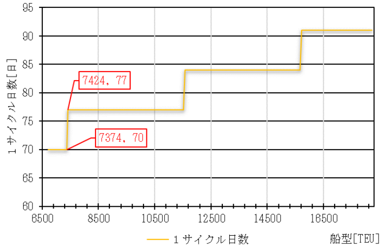
東アジア-北米航路における船型と 1 サイクル日数
