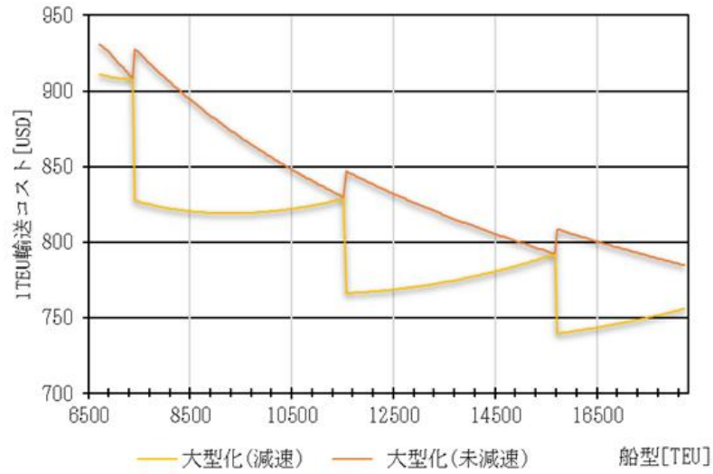
図 5. 2. 1. 10 大型化による隻数増加の減速航海のコスト削減
