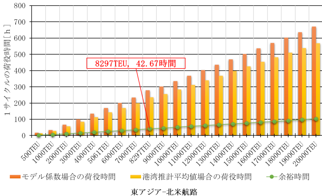
図 5.4.8 東アジア-北米航路の荷役時間の変化
