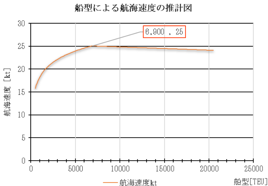
図 4.5.1 平均船型と航海速度の関係
