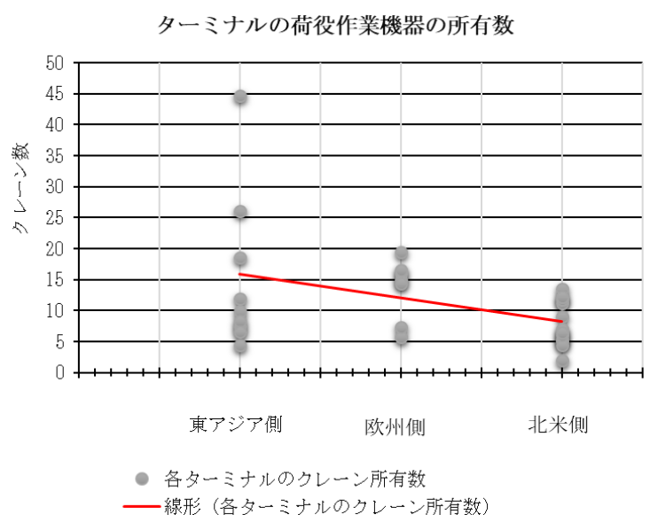
図 5. 4. 3 各地域範囲別のターミナルにおける荷役作業機器の所有数 (26)
