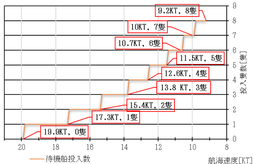
図 5.2.2.2 待機船の投入による減速航海
