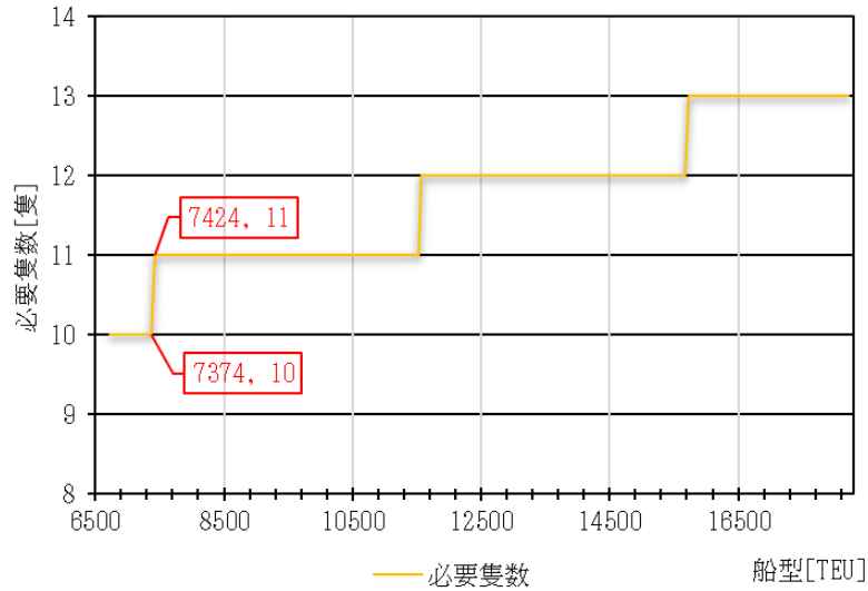
図 5.2.1.3 大型化による必要隻数の変化
